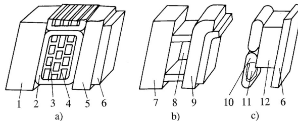
Fig. 3 Exemple de blindaj stratificat
