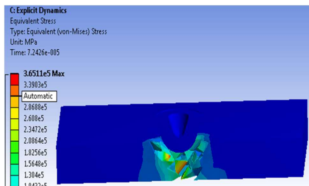
Fig. 19 Tensiunile interne von-Mises
