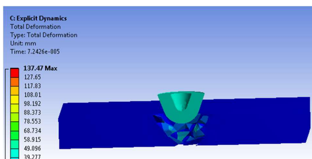
Fig. 18 Deformația totală
